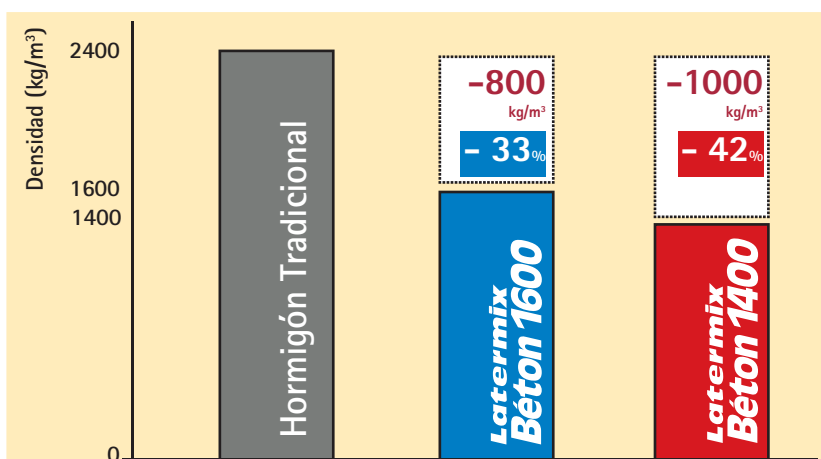
Gama Latermix Beton: Densidades y reducción de las cargas en comparación con el hormigón estructural tradicional.
