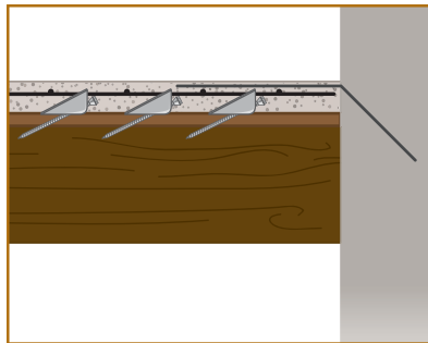
Corte constructivo.
