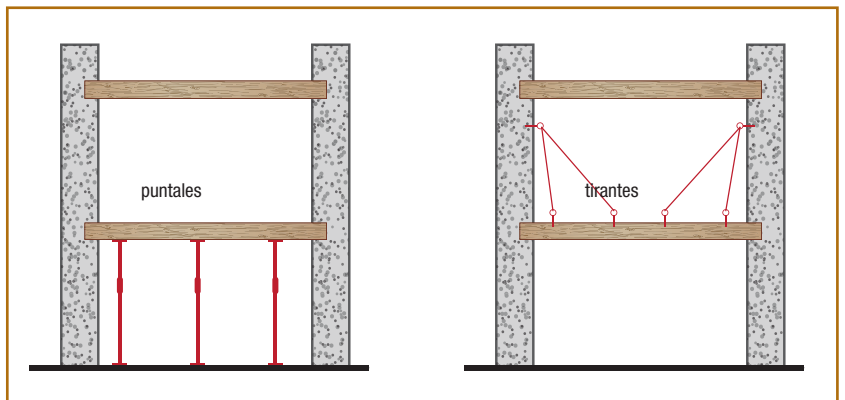
Métodos de apeo del forjado.
