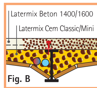
Solución estándar (A) y solución para máxima reducción de cargas (B).
