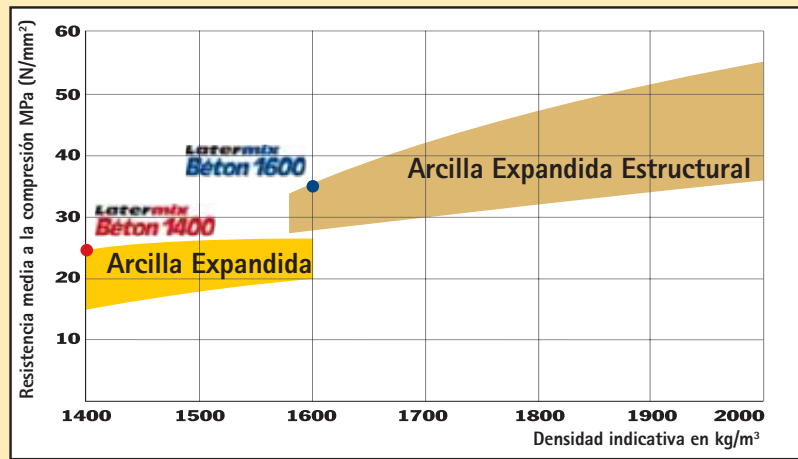
Arcilla Expandida Laterlite Estructural (alta resistencia).
