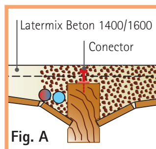
Solución estándar (A) y solución para máxima reducción de cargas (B).
