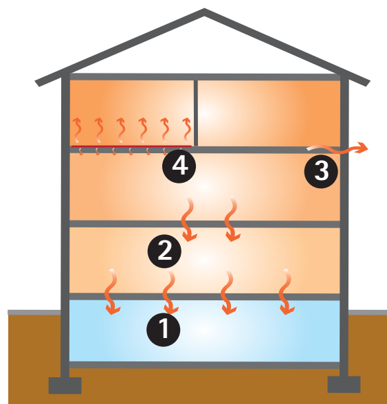
Trasmisión de calor a través de los forjados.
